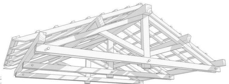
Charpente traditionnelle
